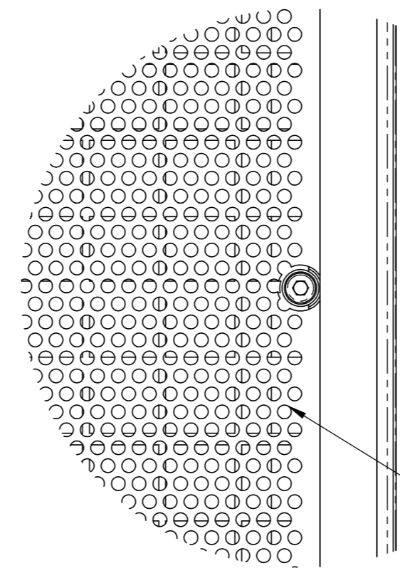
DETAIL C MABSTAB 3 : 7
